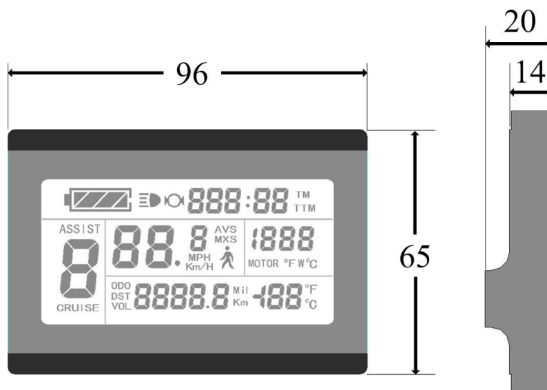
仪表主体外形尺寸
