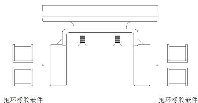
仪表主体和双支架
