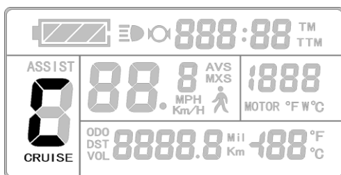
巡航功能 (CRUISE) 显示
