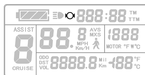
刹车状态显示
