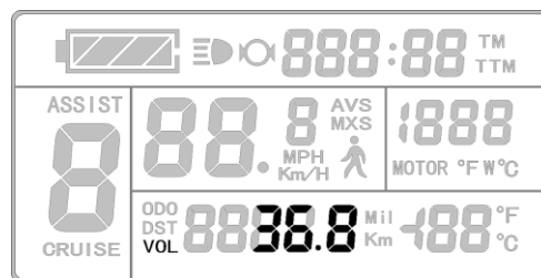
电池实时电压 (VOL) 显示
