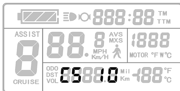
C5参数设置界面
