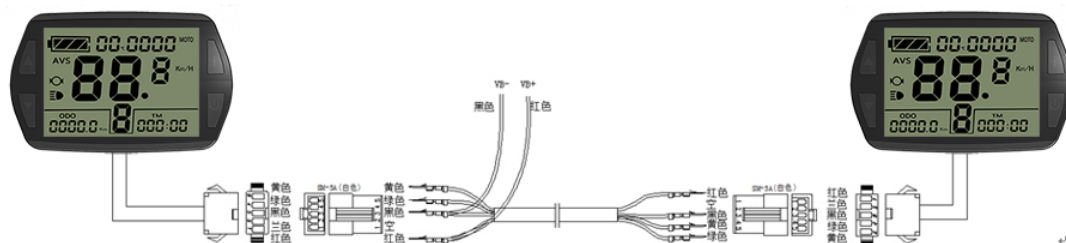
仪表参数复制连线图
