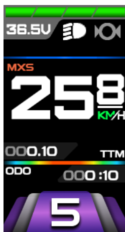
显示界面三
