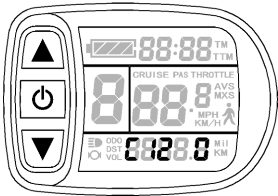
C12参数设置界面
