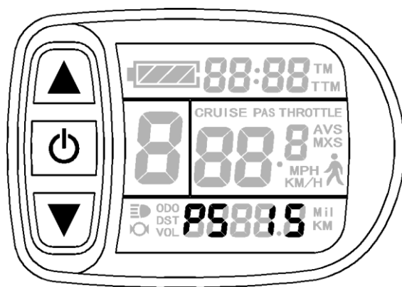
P5 参数设置界面
