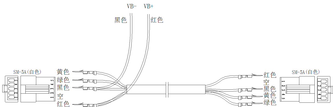
仪表参数复制连线图
