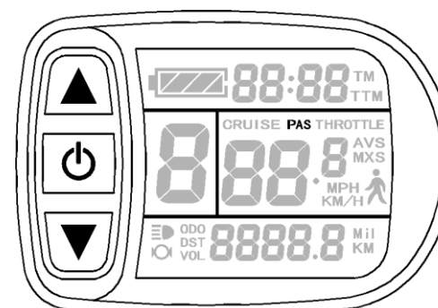
助力启动 (PAS) 显示
