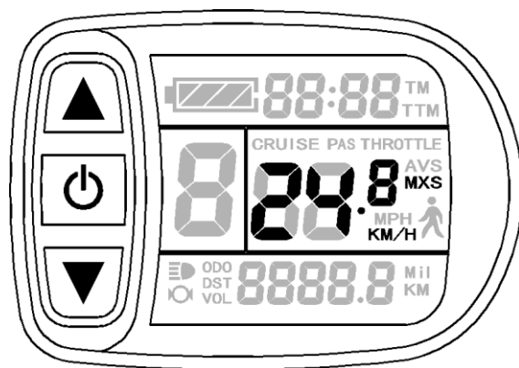
最高骑行速度设置界面
