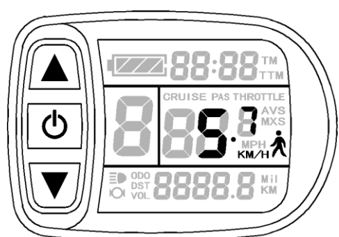
6Km/H助推功能显示
