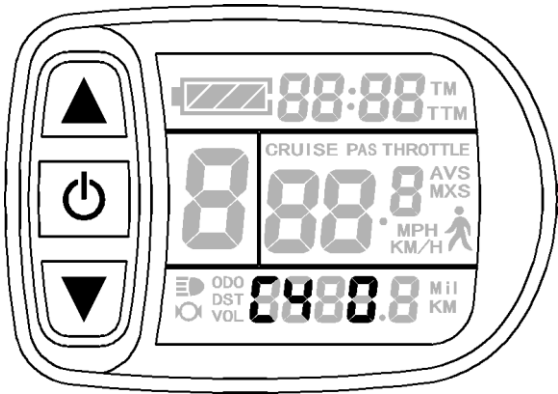
C4参数设置界面
